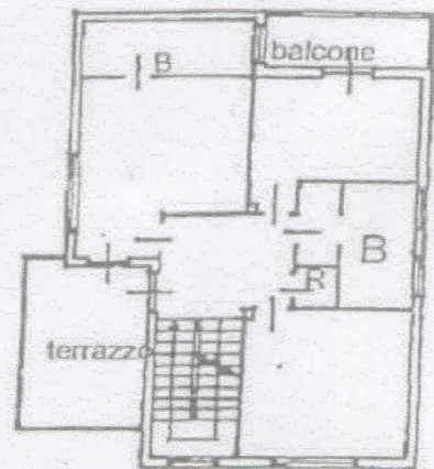
piano primo H=310
